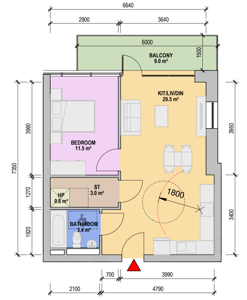
8 APT TYPE - 1H 1 : 100
