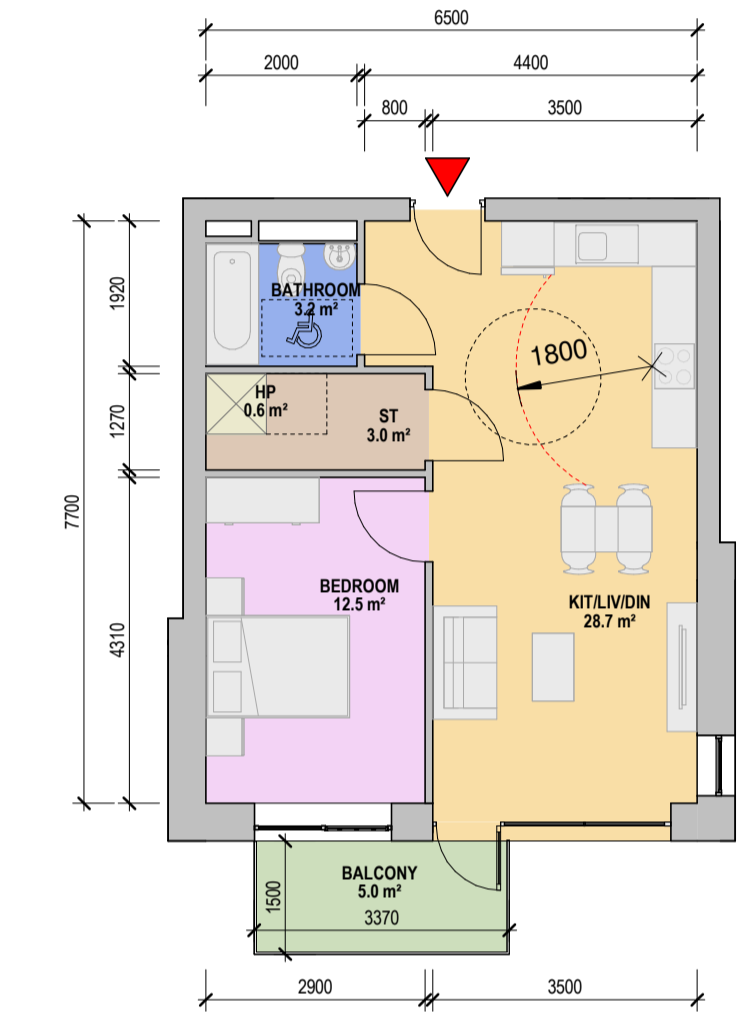
4 APT TYPE - 1D 1 : 100
