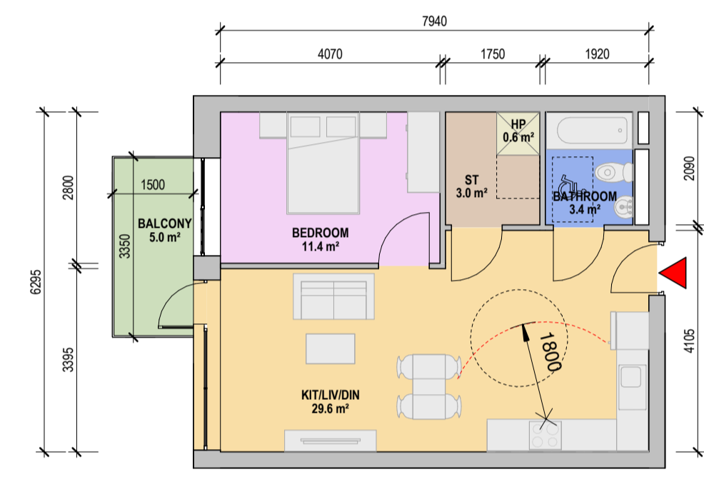
6 APT TYPE - 1F 1 : 100
