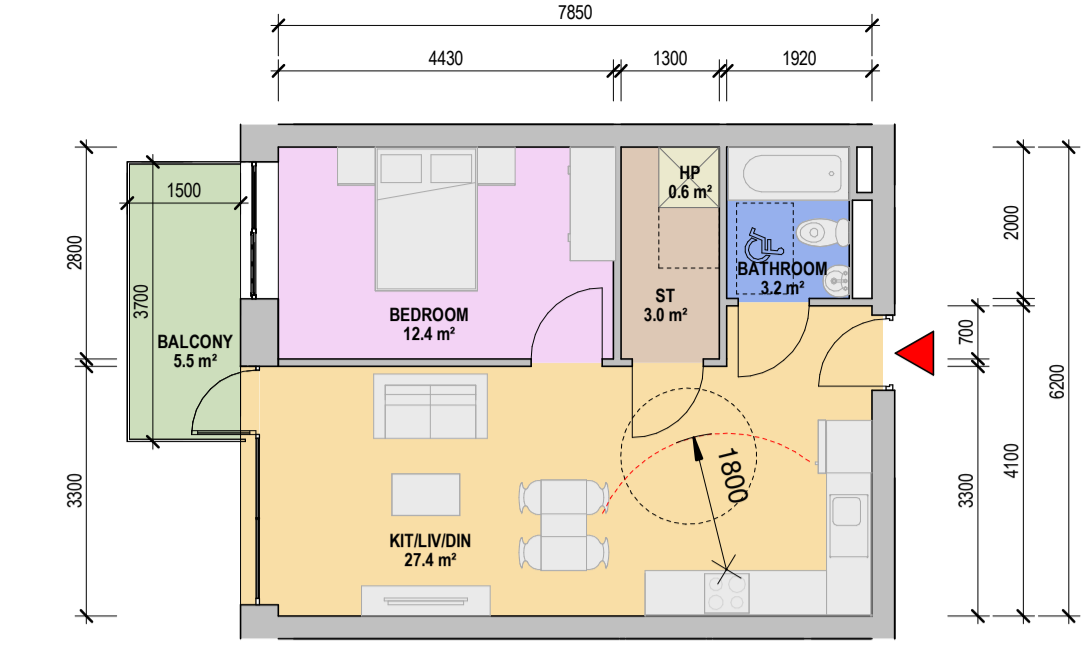
3 APT TYPE - 1C 1 : 100
