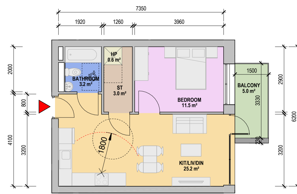
1 APT TYPE - 1A 1 : 100
